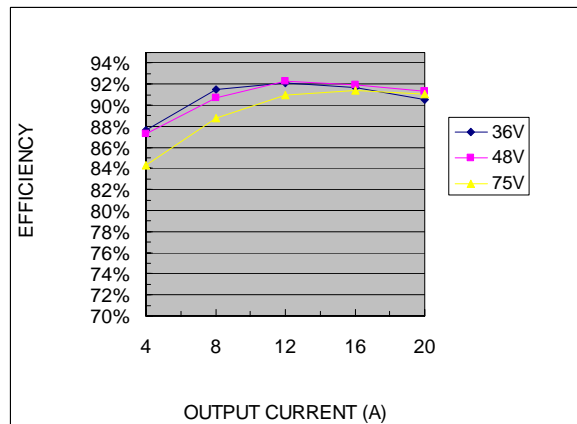
Vo=5V
