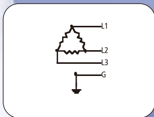
三相; 4线 Delta „Ungrounded“ (3 Ph Δ, 3 W + G) 240 V 480 V
