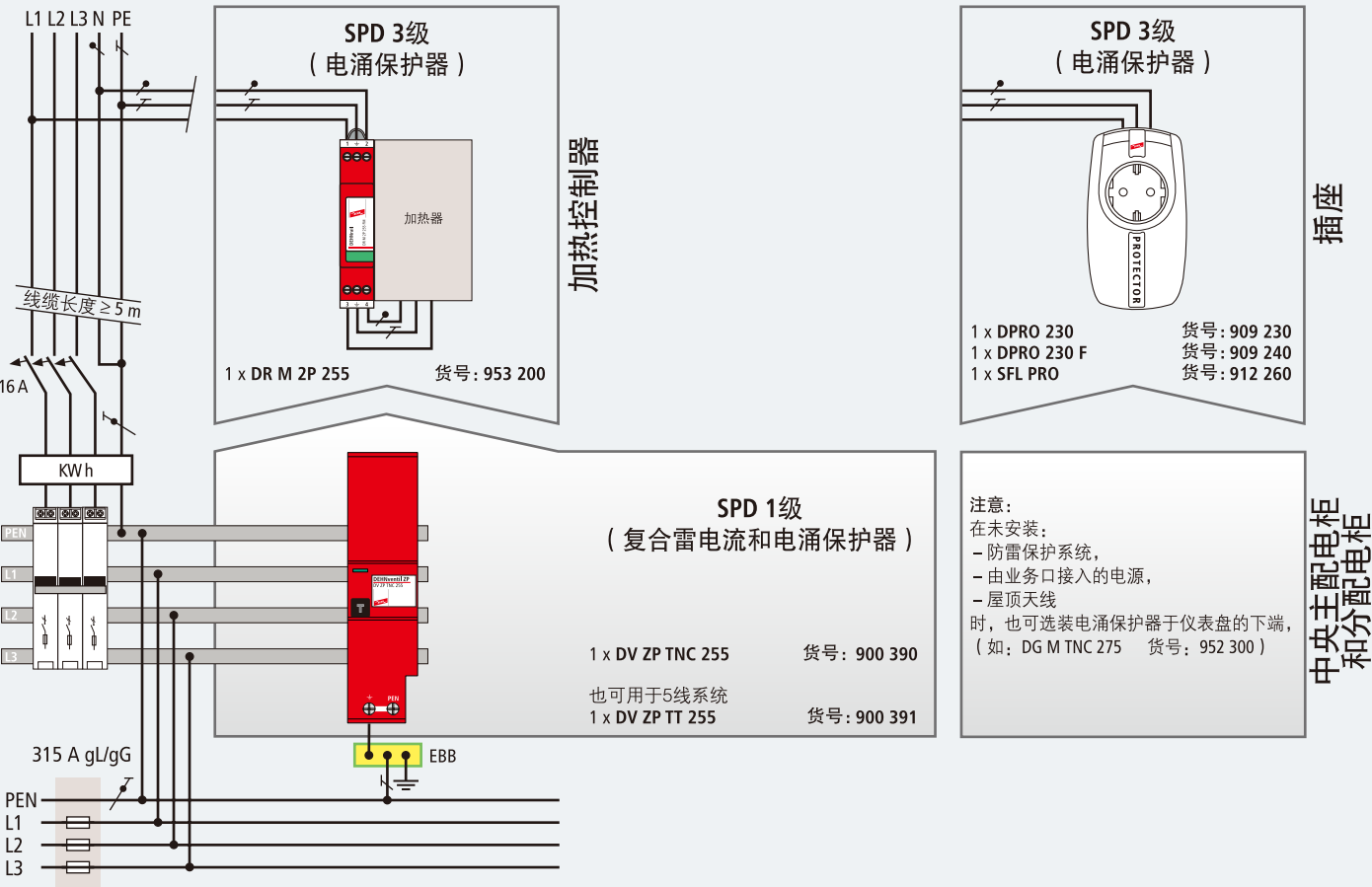
TN 系统: 例子: 住宅楼的保护
