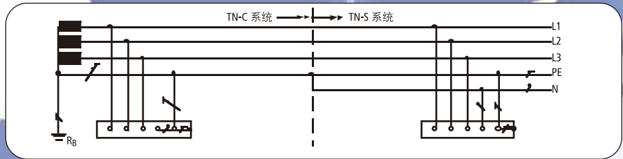
TN-C-S系统 230 / 400 V
