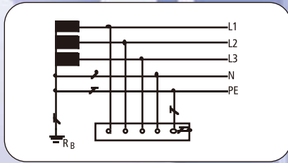
TN-S系统 230 / 400 V
