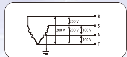
三相; 3线 + 单相; 3线 100 V / 200 V; 200 V
