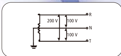
单相; 3线 (1 Ph, 3 W) 100 V / 200 V
