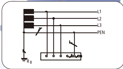
TN-C系统 230 / 400 V
