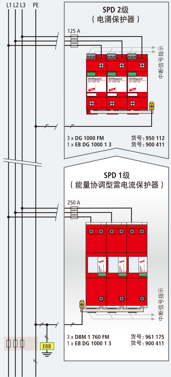
IT 系统：供电制式是690V IT系统，不带中线（N线）。
