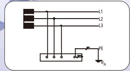
IT-系统 230 V
