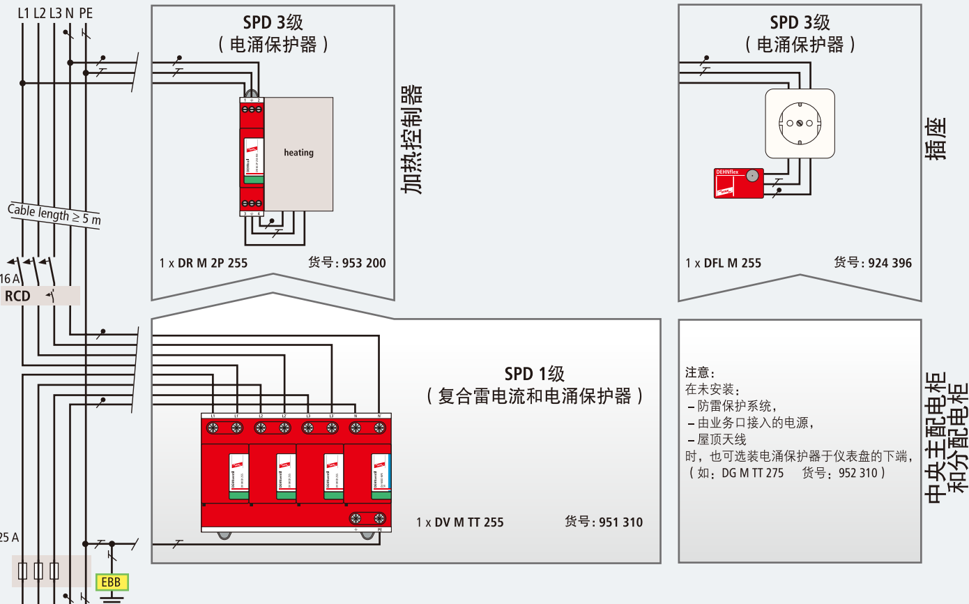
TT 系统: 例子: 住宅楼的保护
