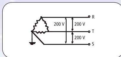
三相; 3线 (3 Ph, 3 W) 200 V
