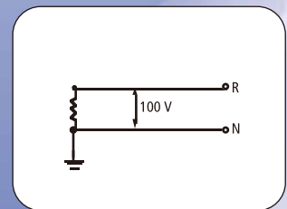
单相; 2线
