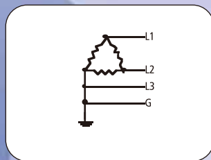
三相; 4线 Delta „Grounded Corner“ (3 Ph Δ, 3 W + G) 240 V 480 V
