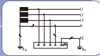
TT系统 230 / 400 V
