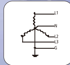
三相; 5线
