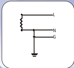
单相; 3线
