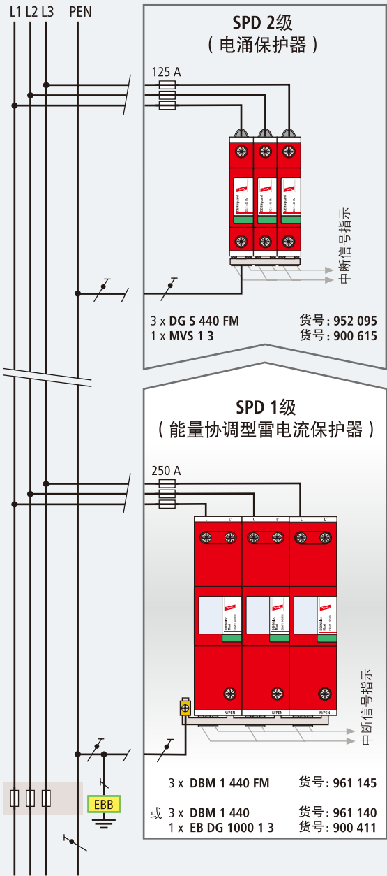
TN 系统：供电制式是400/690V TN-C系统。
