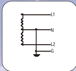
单相; 4线
