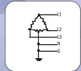
三相; 5线 Delta „Highleg“ (3 Ph Δ, 4 W + G) 120 V / 240 V
